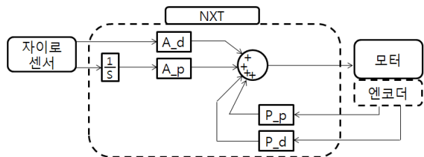
그림 10. 두휠 밸런싱 로봇 제어 블록도 Fig. 10. Control block diagram for two-wheel balancing robot
