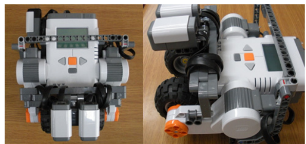
그림 13. NXT를 이용한 투휠 밸런싱 라인트레이서 Fig. 13. Two-wheel balancing line tracer using NXT
