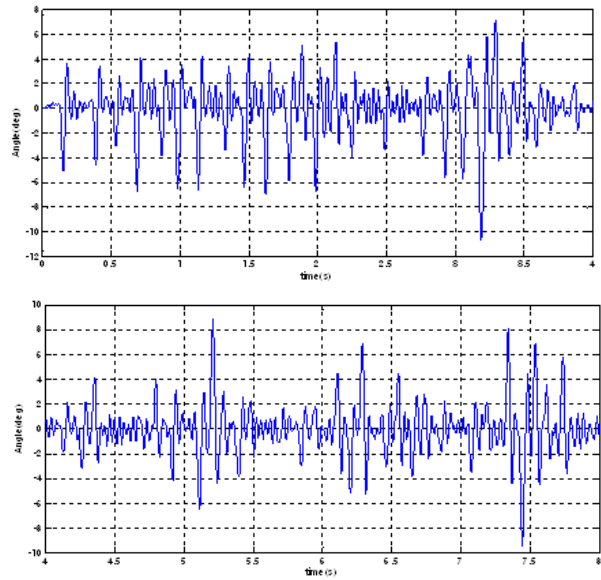
그림 12. 0초에서 8초 까지 자이로 센서 데이터 Fig. 12. Gyro sensor data for 0 to 8 seconds
