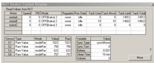
그림 5. Debug windows 프로그램 Fig. 5. Debug window program
