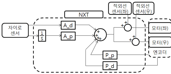
그림 14. 투휠 밸런싱 라인트레이서 제어 블록다이아그램 Fig. 14. Control block diagram for two-wheel balancing line tracer
