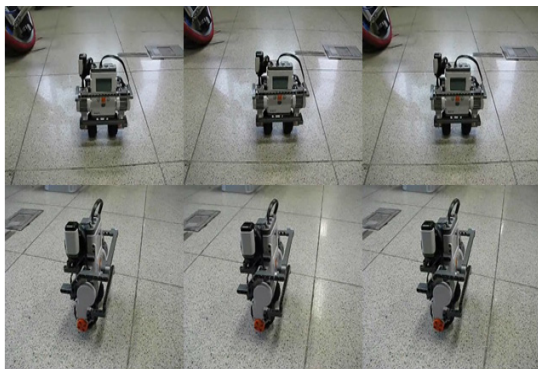
그림 11. 투휠 밸런싱 동영상 Fig. 11. Image cuts of Two-wheel balancing
