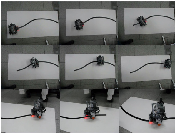
그림 15. 투휠 밸런싱 라인트레이서 동영상 Fig. 15. Image cuts of two-wheel balancing line tracer
